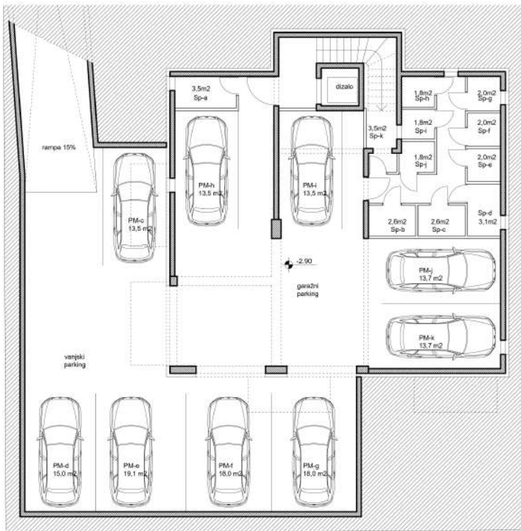
PODRUM - SPREMIŠTA I PARKING MJESTA
