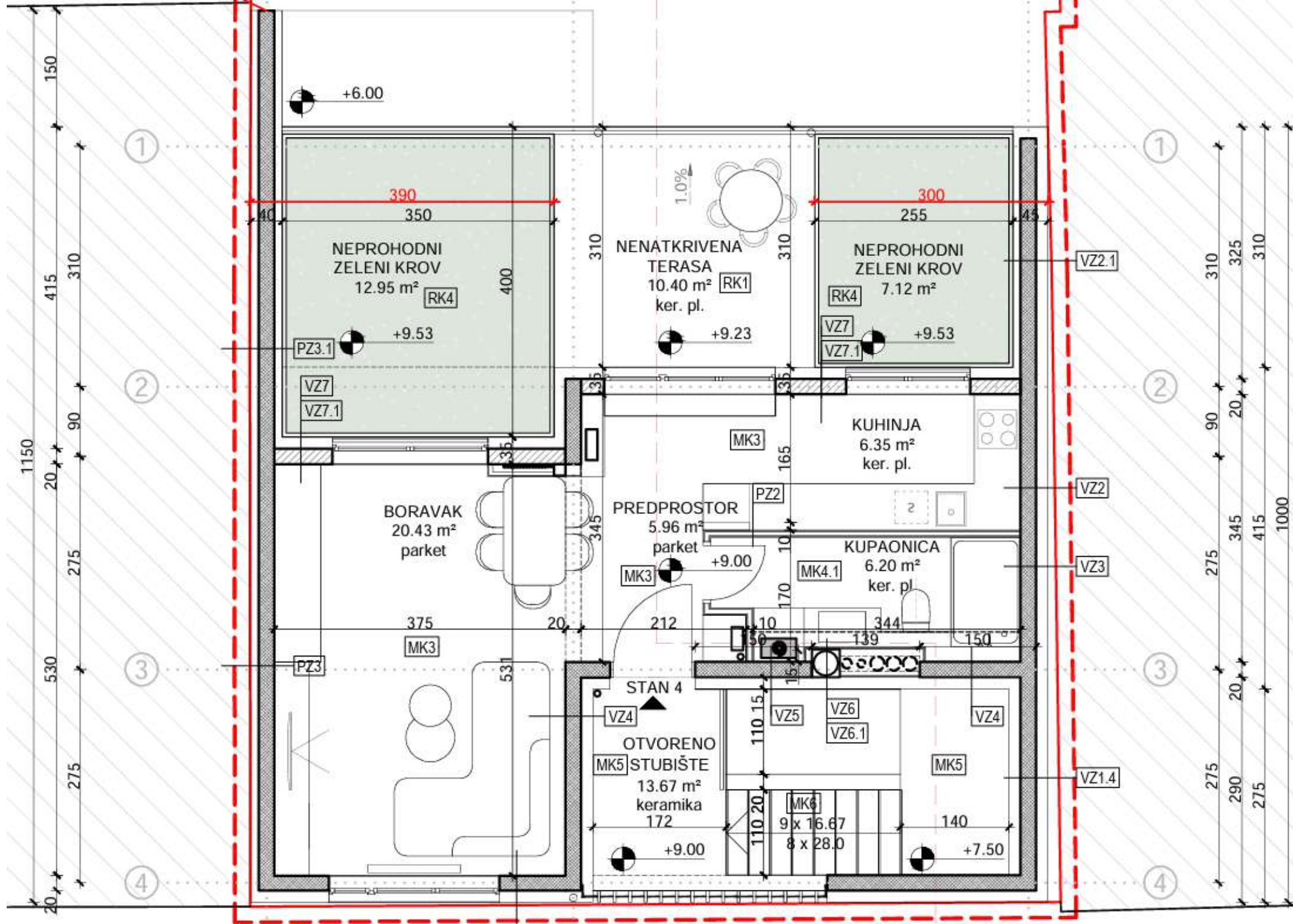
ORIGINALNI TLOCRT 3. KATA
