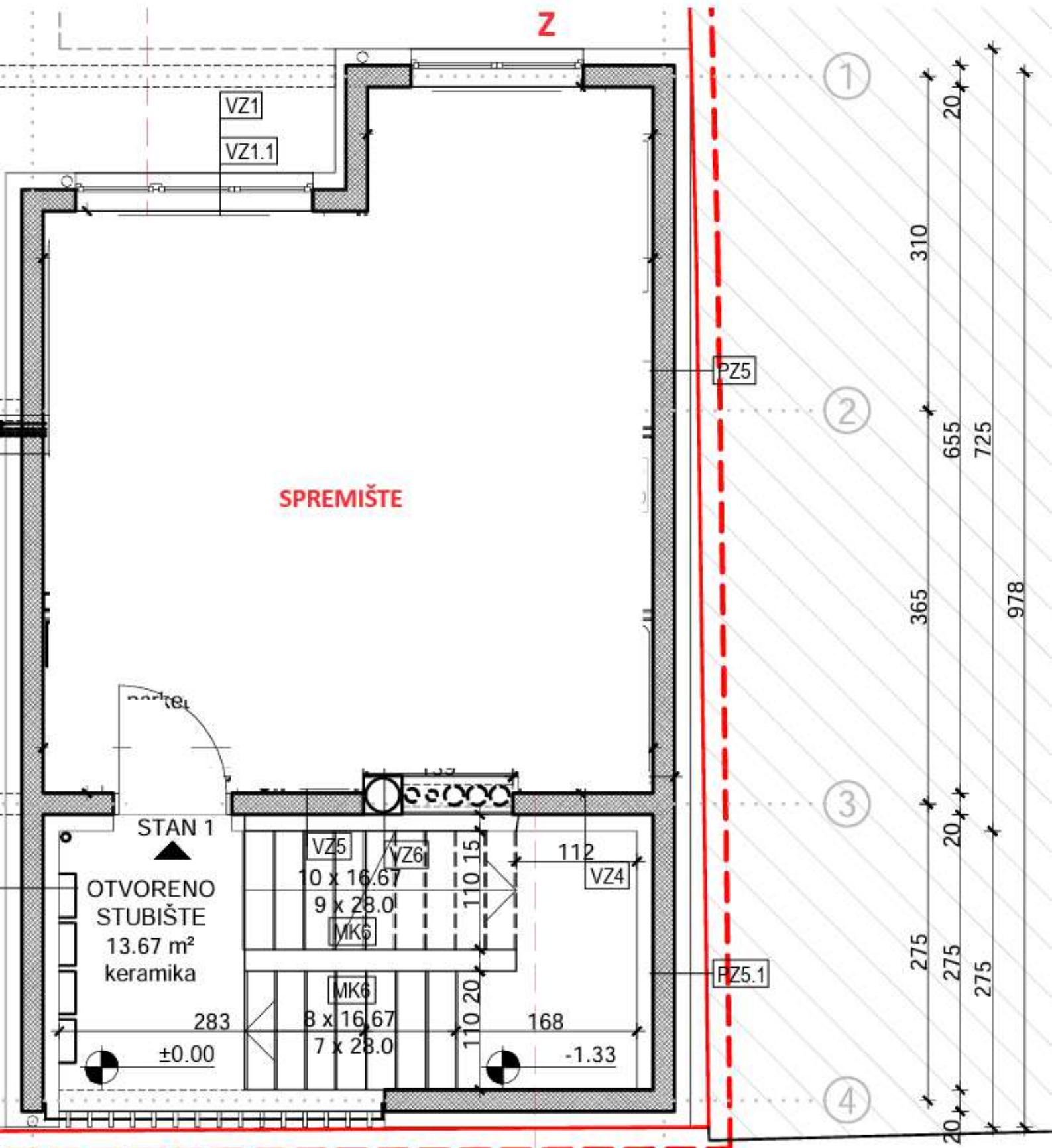
ORIGINALNI TLOCRT PRIZEMLJA
